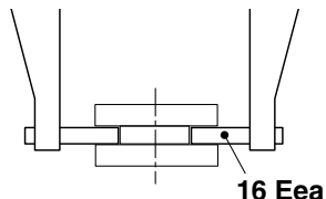
Tapintók külső mérésre
