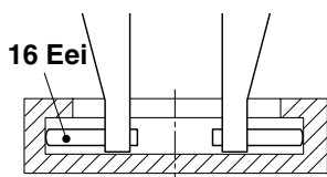
Tapintók belső mérésre
