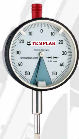
Mérőóra ütésvédelemmel Templar M.S. +0,5 / -0,5 / 0,01mm
